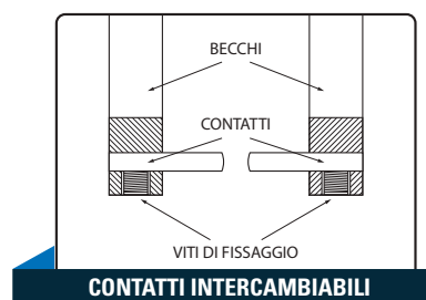
Installazione contatti
